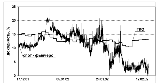
Рис. 4.7. Доходность «spot-фьючерс»
