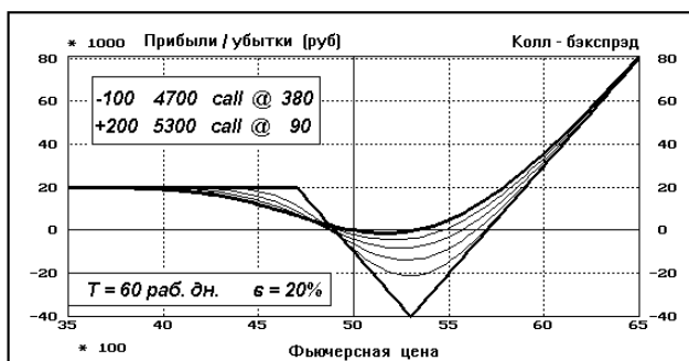
Рис. 11.3. Колл-бэкспред
