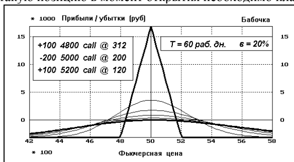
Рис. 11.7. Бабочка
