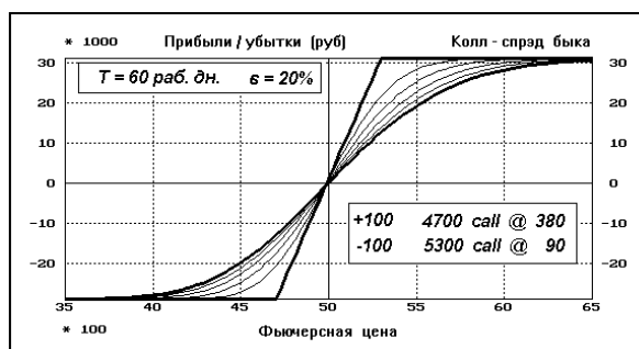
Рис. 11.1. Спред быка
