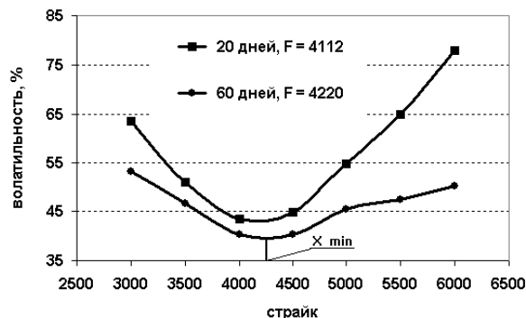
Рис. 10.7. Кривые волатильности
