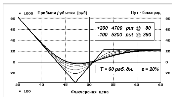
Рис. 11.4. Пут-бэкспред
