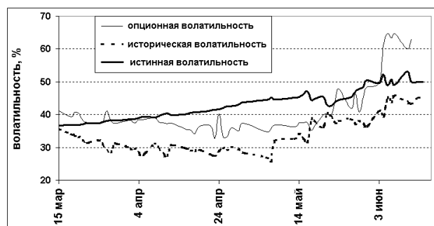
Рис. 10.15. Волатильности
