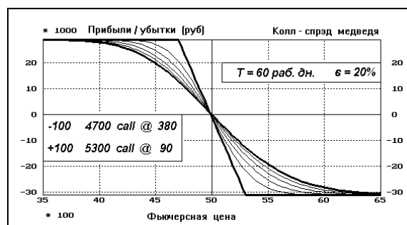
Рис. 11.2. Спред медведя
