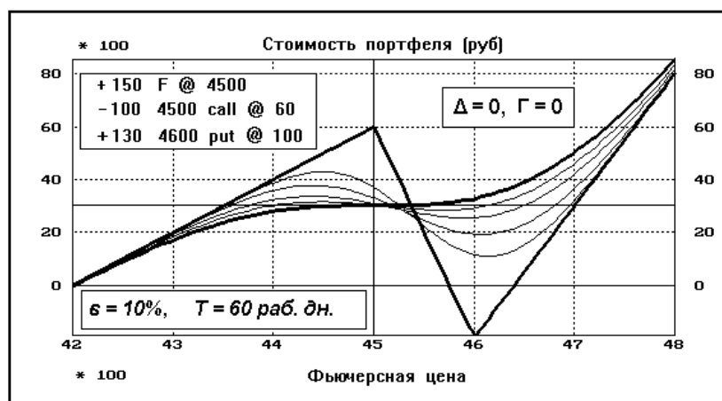
Рис. 9.4. Δ-Γ-нейтральная позиция
