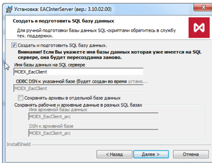
Рис. 7. Мастер установки EACInterServer. Создание базы данных
