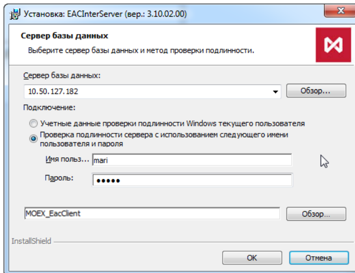
Рис. 11. Мастер установки EACInterServer. Сервер БД
