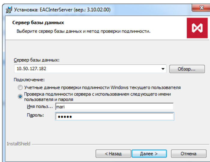
Рис. 8. Мастер установки EACInterServer. Сервер базы данных.
