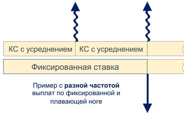
Схема 2. Процентный своп IRS KEYRATE.
